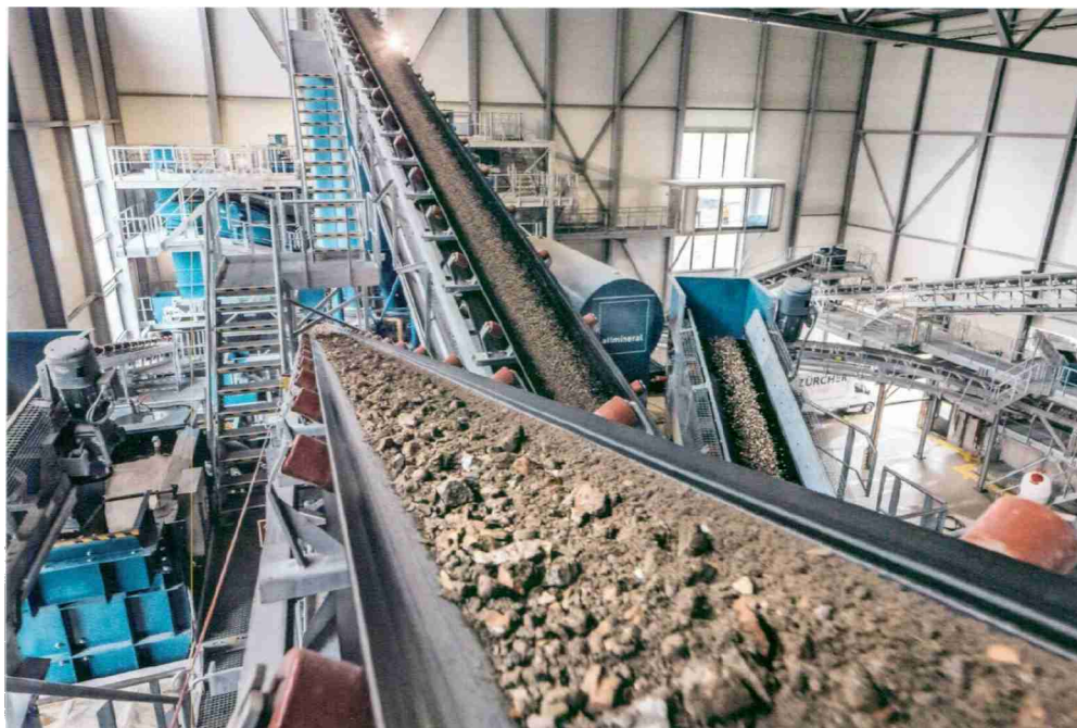
Die Anlage bereitet Rückbaumaterialien wie Misch- und Betonabbruch sowie belastete Aushubmaterialien auf.
